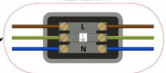
KOBLINGSDIAGRAM
