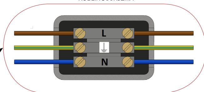
KOBLINGSSKJEMA
