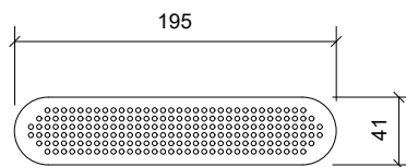
Plan/Plan/Draufsicht
