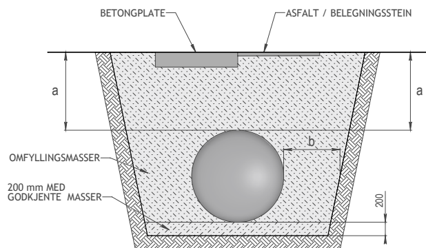
Figur 5: Krav til overdekning.
