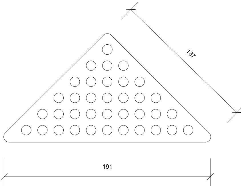
Plan/Plan/Draufsicht
