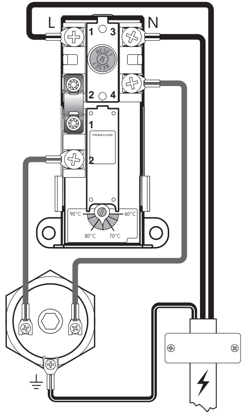
El-kobling, skjematisk
