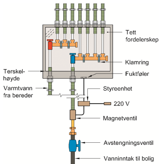
Fig. 5 Fordelerskapp uten drenering, men med lekkasjestopper som stenger vanntilførselen automatisk ved lekkasje
