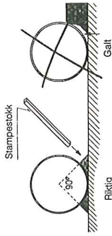
Fig. 2 Pakking av fyllmasse under tankens nederste kvartsirkel
