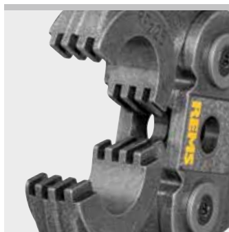
Presstænger med fortdanding forhindrer graddannelse på pressfittingen Patent EP 2 027 971
