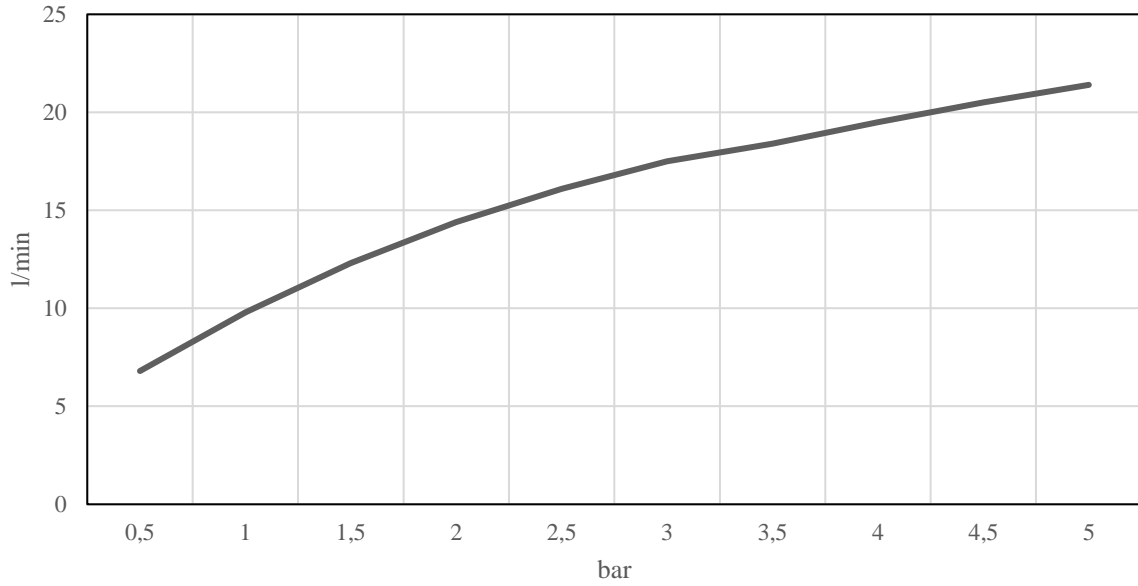
QT1150 flow rate(l/min)
