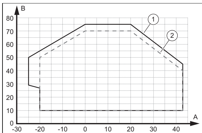
A Udetemperatur B Anlægsvandtemperatur 1 Anvendelsesgrænser, normaldrift, opvarmning 2 Anvendelsesgrænser, startfase, opvarmning
