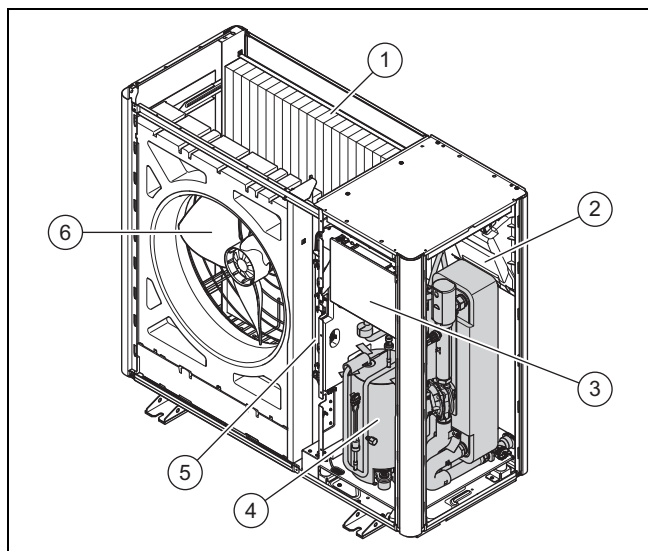
1 Fordamper 4 Kompressorkomponenter 2 Printplade INSTALLER BOARD 5 Komponenter INVERTER 3 Printplade HMU 6 Blæser
