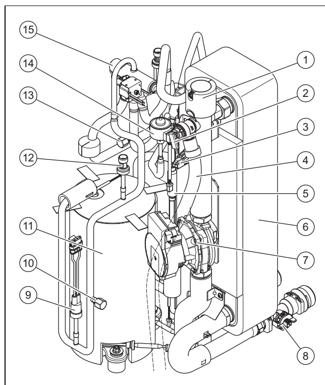
1 Automatudluffer 9 Trykvagt, i højtryksområdet 2 Sikkerhedsventil 10 Vedligeholdelsestilslutning, i højtryksområdet 3 Trykføler i varmekredsen 11 Kompressor 4 Afløbsslange sikkerhedsventil 12 Trykføler, i højtryksområdet 5 Filter 13 Vedligeholdelsestilslutning, i lavtryksområdet 6 Kondensator 14 Elektronisk ekspansionsventil 7 Varmepumpe 15 4-vejsomskifterventil 8 Gennemstrømningsføler
