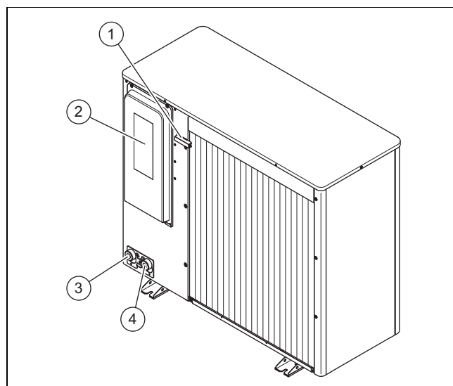
1 Temperatursensor, ved luftindgang 3 Tilslutning til varmeanlæggets returløb, G 1 1/4" 2 Elektriske tilslutningers afdækning 4 Tilslutning til varmeanlæggets fremløb, G 1 1/4"
