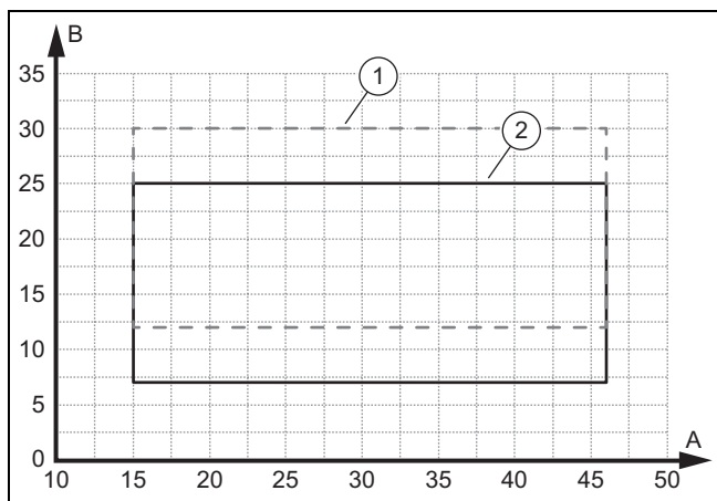
A Udetemperatur B Anlægsvandtemperatur 1 Anvendelsesgrænser, startfase, køling 2 Anvendelsesgrænser, normaldrift, køling
