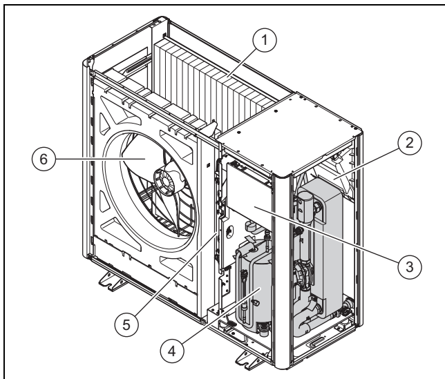
1 Luftutløpsgitter
