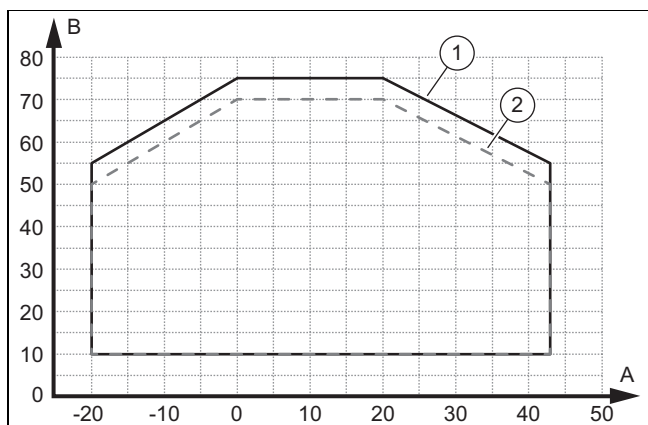
A Udetemperatur B Anlægsvandtemperatur 1 Anvendelsesgrænser, normaldrift, varmtvand 2 Anvendelsesgrænser, startfase, varmtvand
