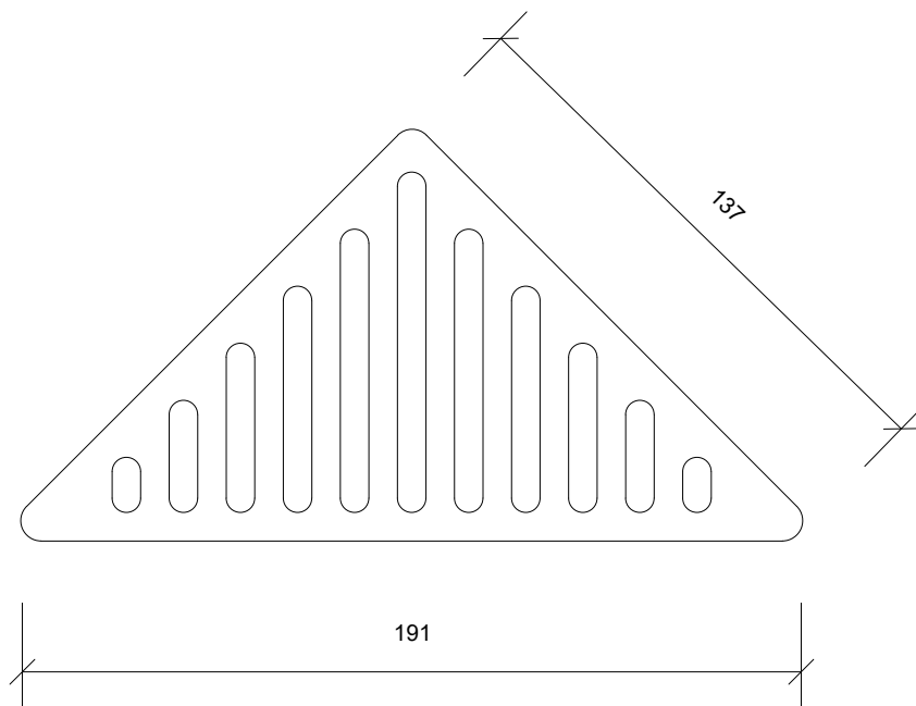
Plan/Plan/Draufsicht
