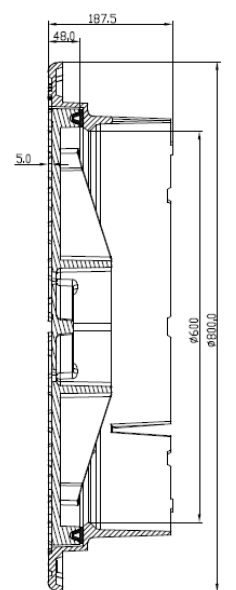
SECTION A-A
