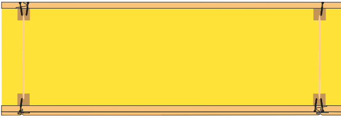
Fig 6.1. Konstruktion bestående av 22 mm Forestia Golv, Masonite Beams I-balk, mineralull, 22 mm Forestia Golv och Tak-ess
