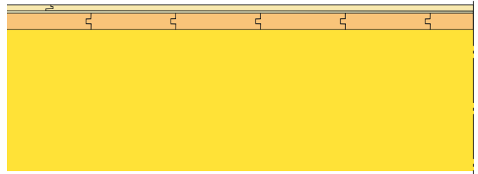
Fig 8.1. Konstruktion bestående av 22 mm Forestia Golv, Masonite Beams I-balk, mineralull, 22 mm Forestia Golv och Tak-ess.
