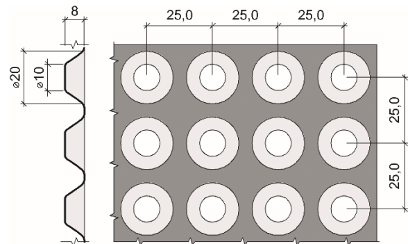
Fig. 1 Jackon DrainPro. Angitt mål i mm.
