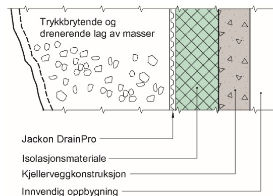
Fig. 2 Bruk av Jackon DrainPro fuktsperre på isolert vegg mot terreng. For raskere uttørking anbefales at Jackon DrainPro fuktsperre plasseres utenpå dampåpen varmeisolasjon som f.eks. EPS, se Byggforskerien 523.111 Yttervegger mot terreng. Varmeisolering og tetting.
