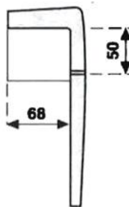
Snitt A-A
