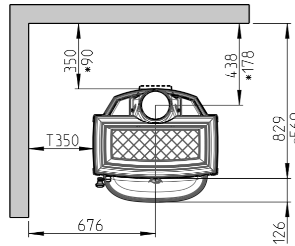
Minimum avstand til brennbar vegg
