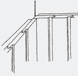
Stående panel innvendig hjørne
