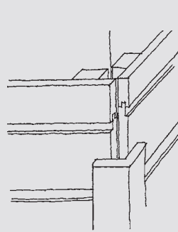
Liggende utvendig hjørne med vinkellist
