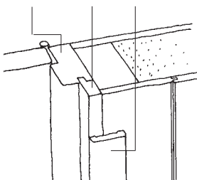
Karm Utføring Karmlist
