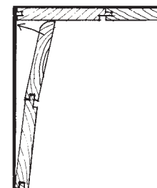
Avslutning mot hjørne (uten hjørnekasse)
