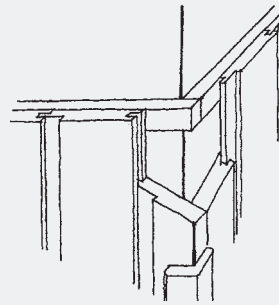
Stående panel, utvendig hjørne med hjørnelist
