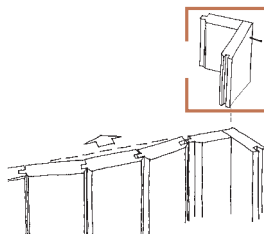
Avslutning mot hjørne (innvendig hjørnekasse spikres/limes)
