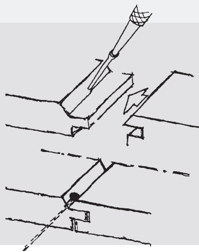
Spikerlengde, ca. 3 x paneltykkelse. Spikertykkelse, minimum 1,6 mm
