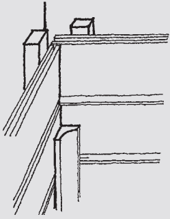
Liggende innvendig hjørne med hulkillist
