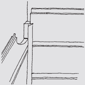
Liggende panel, innvendig hjørne, med vår spesial hjørnelist
