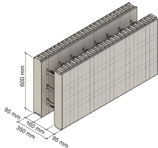
Fig. 1 Vartdal Blokk Standard (mål i mm)
