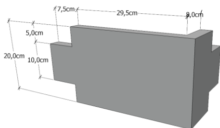
UTVENDIG HJØRNE SC 44
