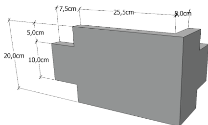
UTVENDIG HJØRNE SC 40
