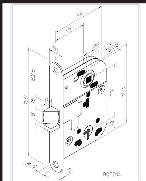
Mål på låskassen (mm)
