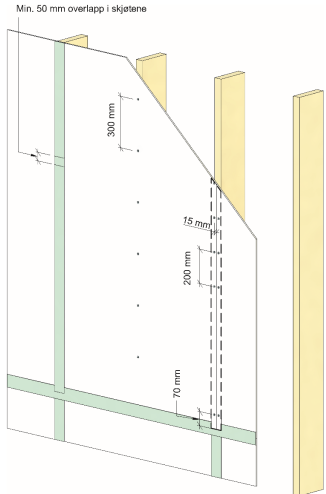
Fig. 1 Cembrit Windstopper montert på yttervegg med trestendere med tape over alle plateskjøtene.
