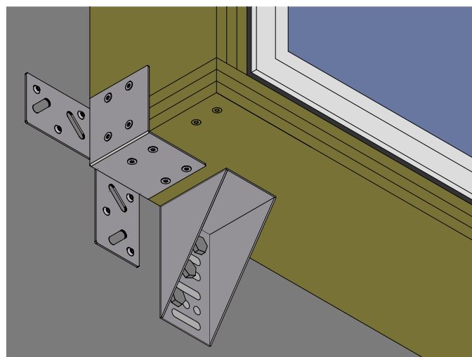
Vinkelbeslag monteres under bunnplaten og plasseres ift beskrivelse på forrige side.
