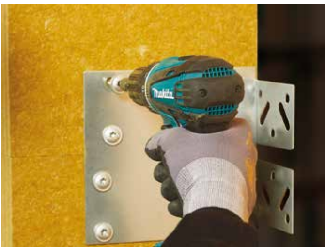
ES/EL skjøtebeslag ved plateskjøter
