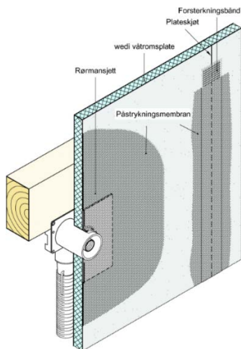
Fig. 3 Prinsipp for vannetting rundt rørgjennomføringer og over skjøter
