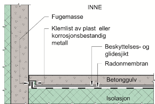
Fig. 2 Eksempel på bruk av RMB 400 Radonsperre i bruksgruppe B. Golv på grunnen med ringmur og betongvegg.
