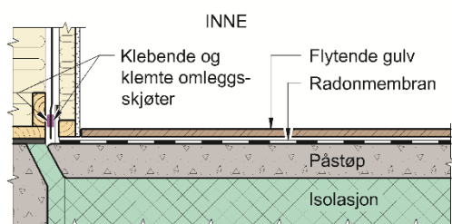
Fig. 3 Eksempel på bruk i bruksgruppe C. Golv på grunnen med ringmur.
