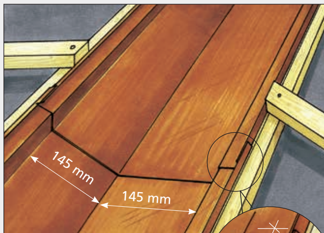
6.3.1 A Powertekk Takfotbeslag Powertekkplatene kan festes på vanlig måte.
