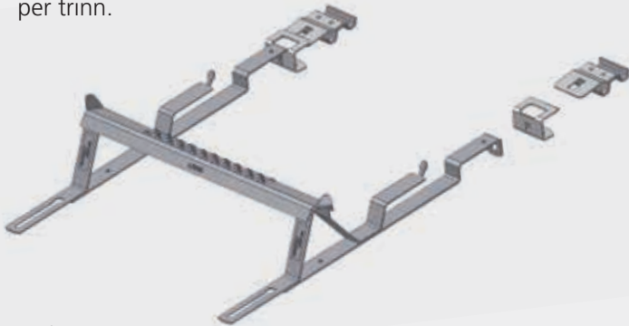
7.10.1.1 A Stigetrinn og 2-delt innfestebøyle
