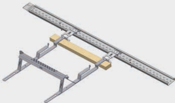
7.10.1.1 B Stigetrinn, 2-delt innfestebøyle og innfesteskinne
