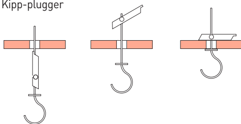
Kipp-plugger
