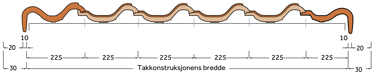
Figur 14: Hollander V med gavlstien
