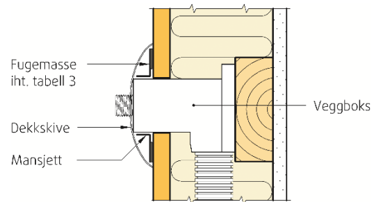
Fig. 3 Rørgjennomføring hvor mansjettens limes fast til baderomspanelet
