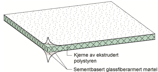
Fig. 1 Oppbygningen av Tetti Våtromsplate. Platen er symmetrisk med armert mørtel på begge sider
