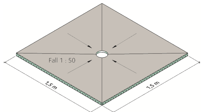
Fig. 2 Eksempel på wedi Fundo gulvelementer med punktavløp sentrert plassert
