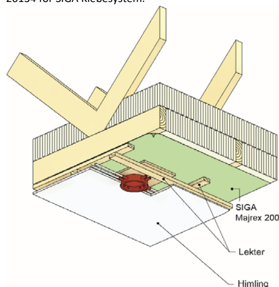
Fig. 3 SIGA Majrex 200 montert i isolert undergurt mot kaldt loft med gipsplate
