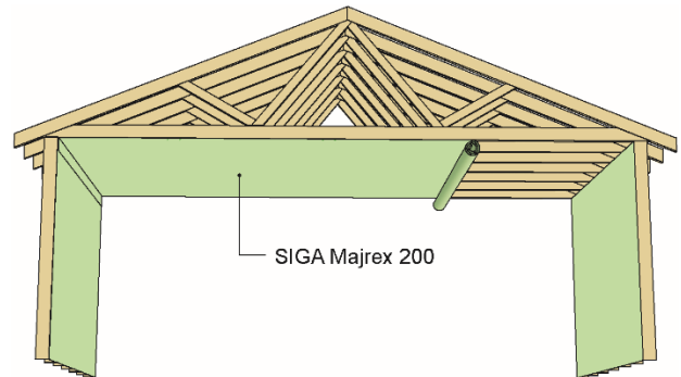
Fig. 1 SIGA Majrex 200 monterert i yttervegg og mot kaldt loftsrom
