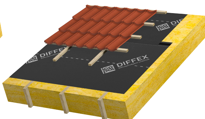
Luftet konstruksjon med AeroDek Tradition Plus på Icopal Ventex Undertak Pro, diffusjonsåpent undertak lagt rett på taksperrene
