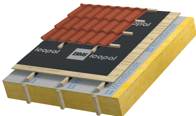
AeroDek Tradition Plus på bærende undertak, tekket med Icopal Underlag Pro underlagsbelegg
