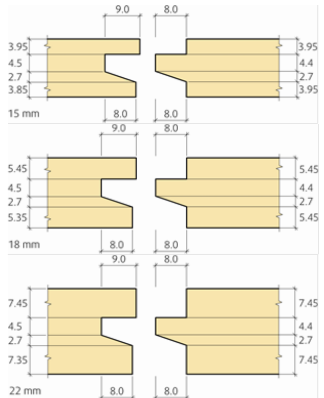
Fig. 1 Krysslaminert massivtreelement
