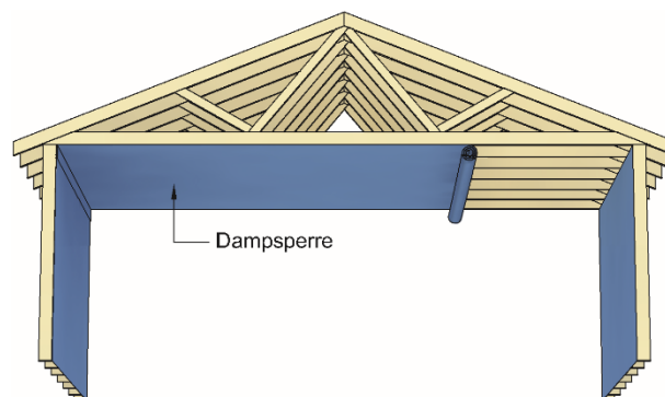
Fig. 1 Glava Dampsperre monterert i yttervegger og mot kaldt loftstom
