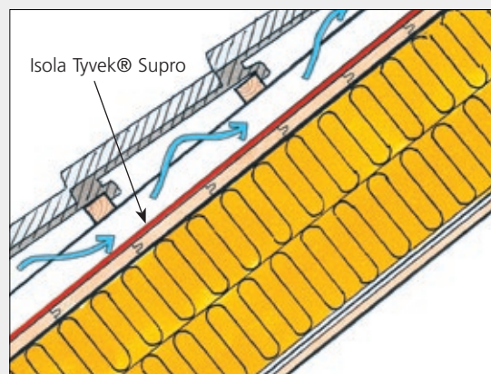
Principskiss av diffusionsöppen konstruktion.
