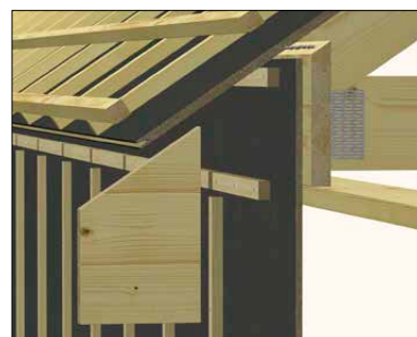
Overgang vegg/tak med løst utstikk
