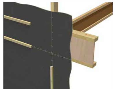
Klemming av skjøter
