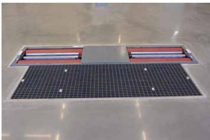
MAHA Eurosystem PC-basert bremsetester godkjent av Volkswagen.
