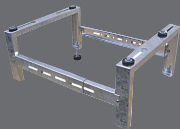
Galvanisert bakkestativ Leveres med vibrasjonsdempere
