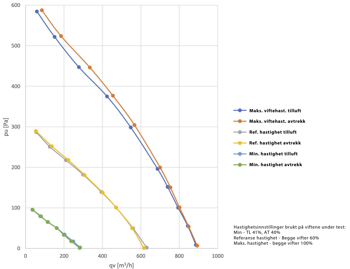
Diagram luftmengde/trykk
