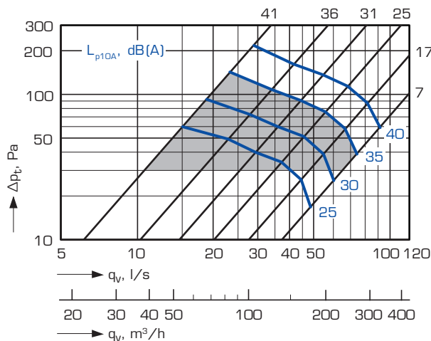
LUMO-200
