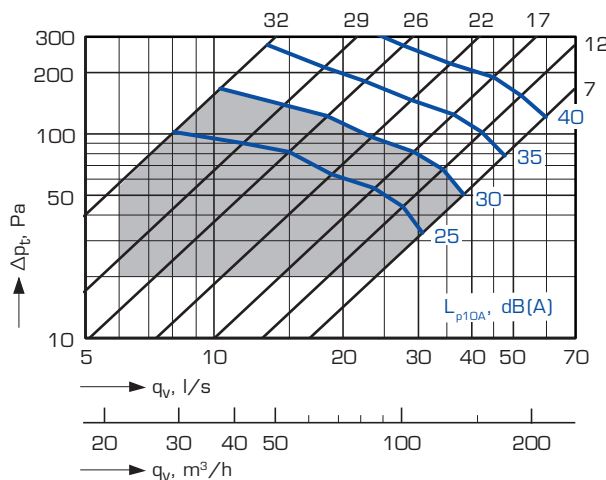
LUMO-125
